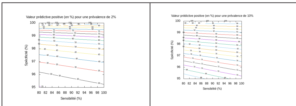
Figure C1.2 Valeur prédictive positive en fonction du couple sensibilité-spécificité.
